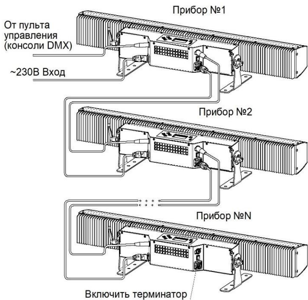
Рисунок 6 – Подключение приборов в линию
