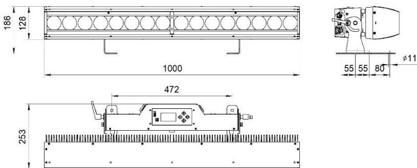
Рисунок 1 ГАБАРИТНЫЕ РАЗМЕРЫ
