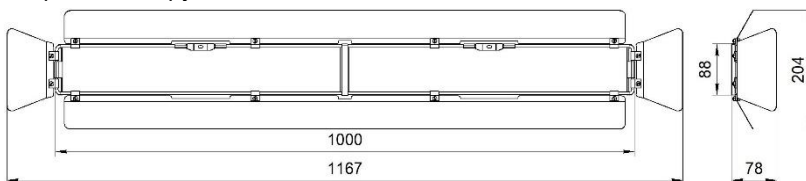
Рисунок 3 Шторки кашетирующие
