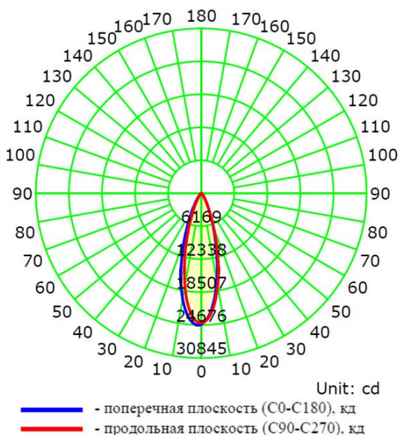
Рисунок 2 Кривая распределения силы света.
