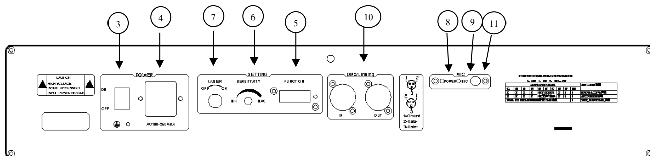
Задняя панель
