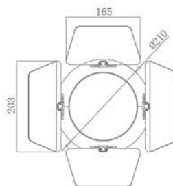
Barn doors (X40482)
