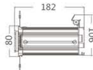
Zoom barrel(19°-36°) (X40291)
