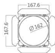
Barn doors (X40029)
